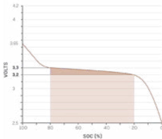
Abbildung 2 - Entladung einer LFP-Batterie / Ladezustands-Berechnung
