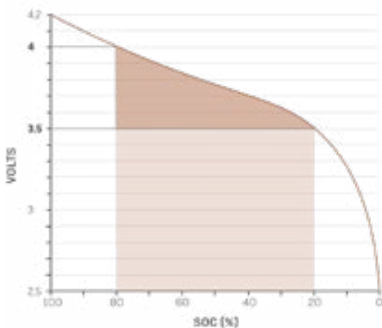
Abbildung 1 - Entladung einer NMC-Batterie / Ladezustands-Berechnung
